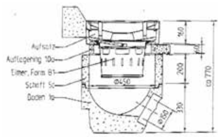
Straßenablauf DIN 4052 Boden 1a, Schacht 5c, Eimer Form B1, Ring 10a, Betonguss-Aufsatz 500 x 500
